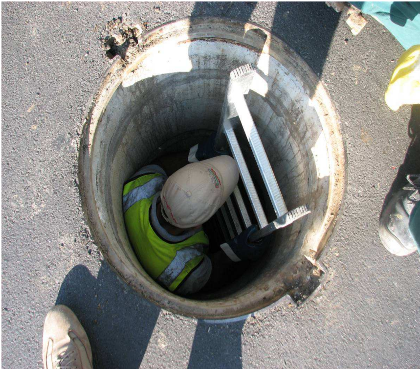
Fig. 1. Esempio reale. Un operatore scende in fogna di acque bianche per orientare una telecamera per video ispezioni. Risulta evidente la non sufficienza dell'allestimento sia per le dimensioni sia per l'impossibilità del recupero dell'infortunato (per gentile concessione di uno degli autori).
